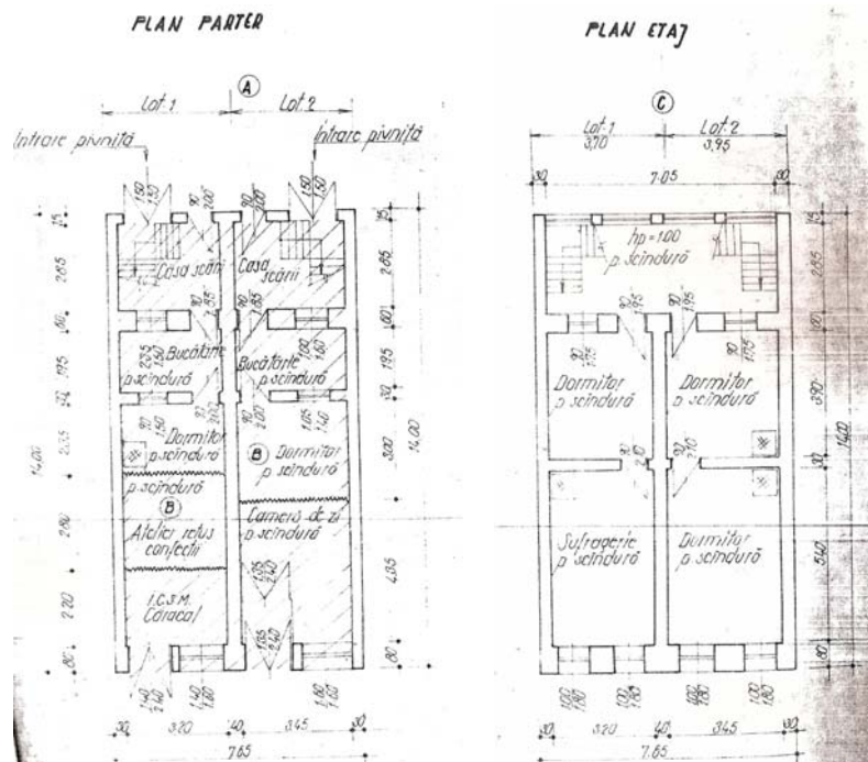
Locuința lui Moscovici Giugea – plan parter și etaj
